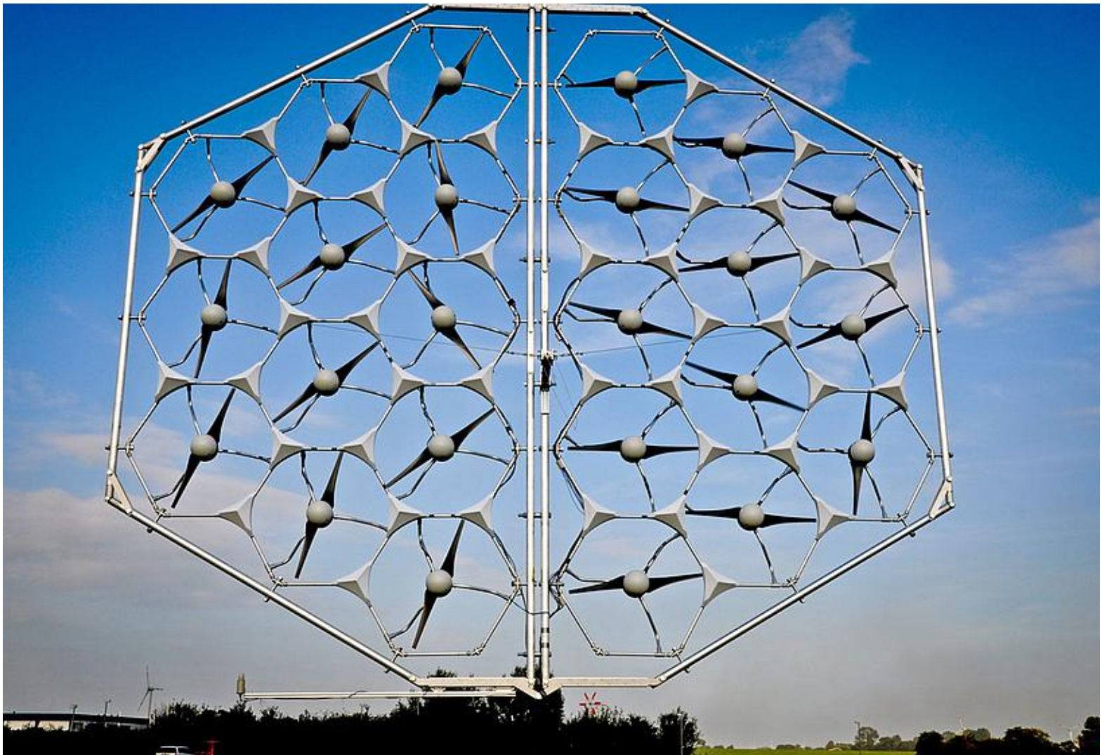
Zusammengeschaltete MOWEA-Windturbinen. (Foto: © MOWEA)
